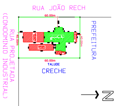
PLANTA SITUAÇÃO ESC: 1/750
