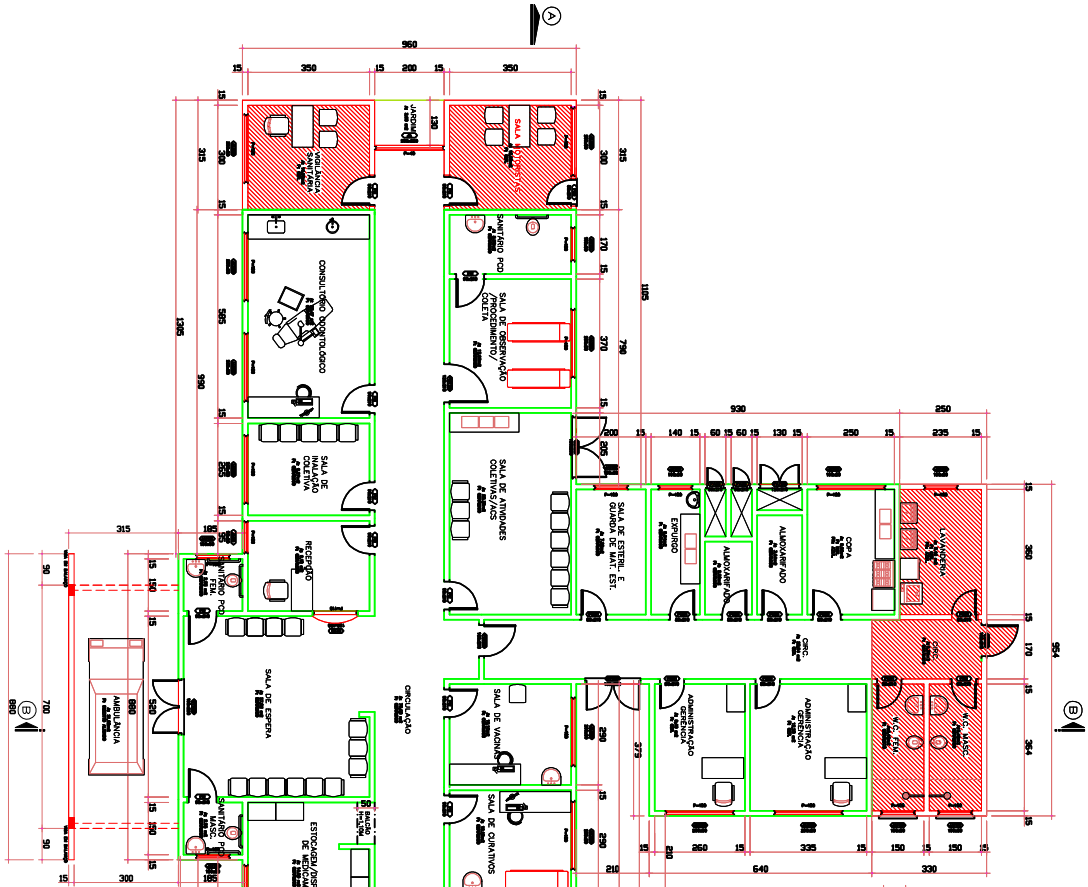
PLANTA BAIXA AREA= 642,53m 2 ESC=1/75
