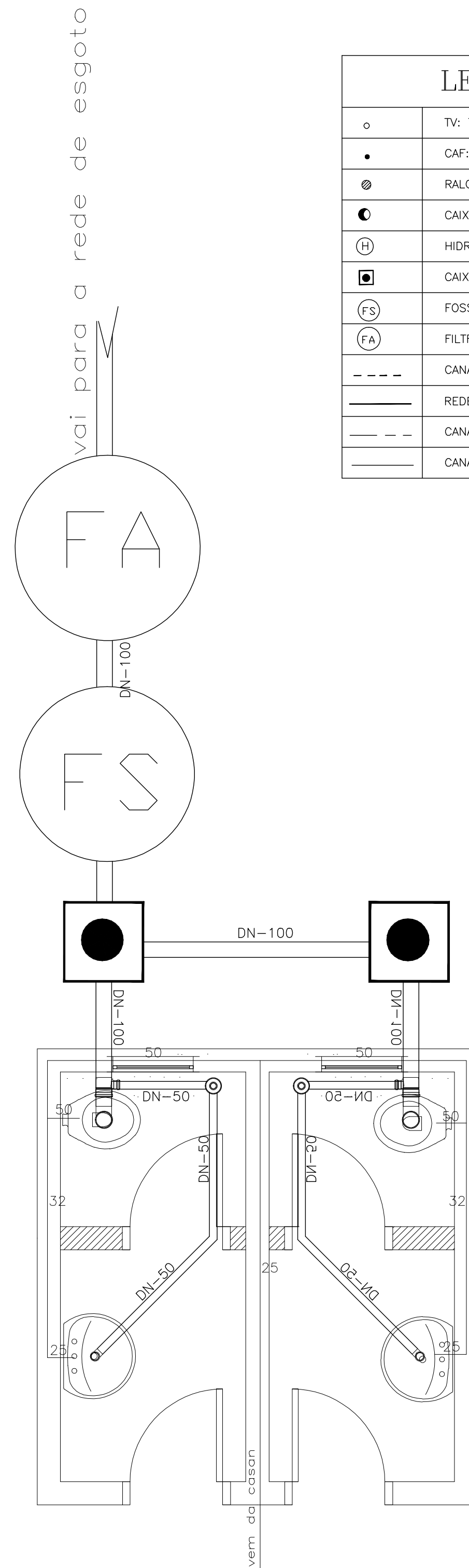
PLANTA HIDROSSANITÁRIO Escala 1/25
