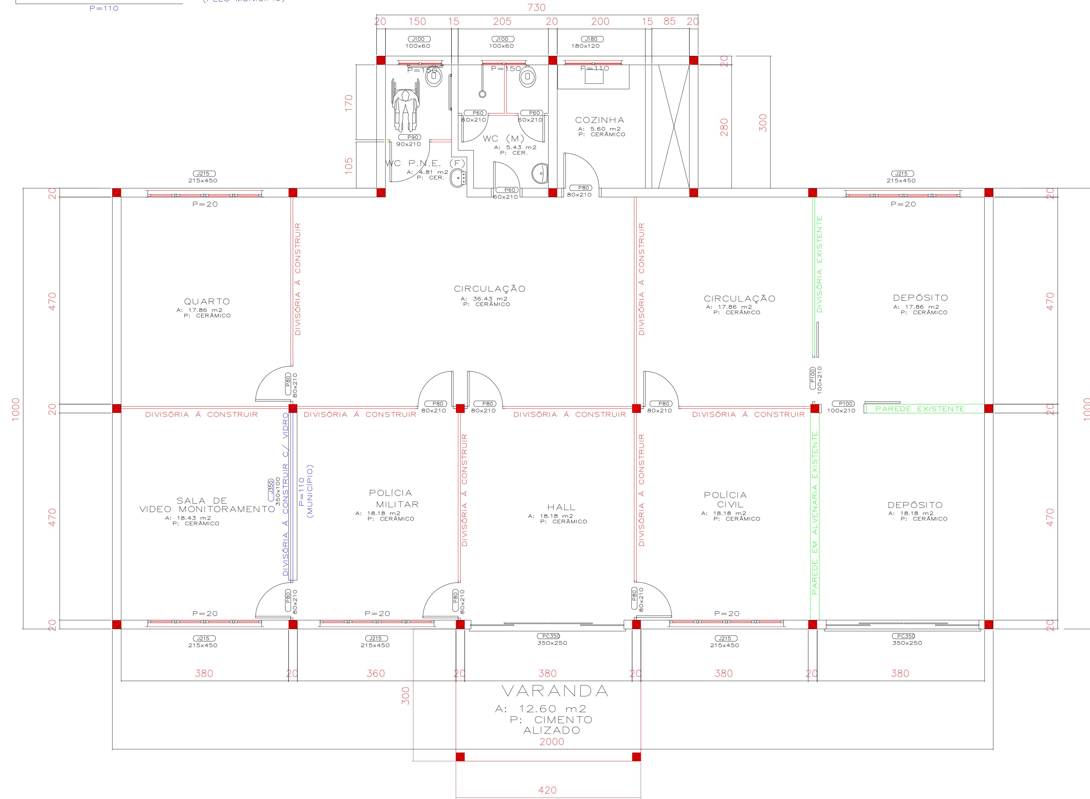
PLANTA BAIXA A: 233,60 m 2 ESC: 1/50
