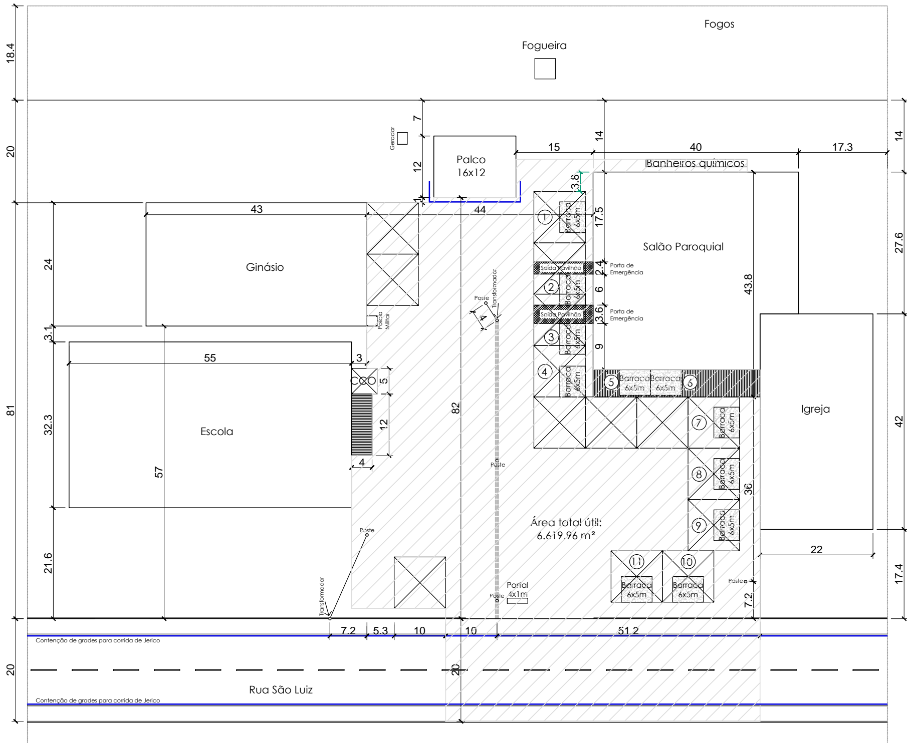
PLANTA DE LOCAÇÃO Sem Escala
