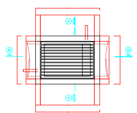
PLANTA BOCA-DE-LOBO Esc. 1/10
