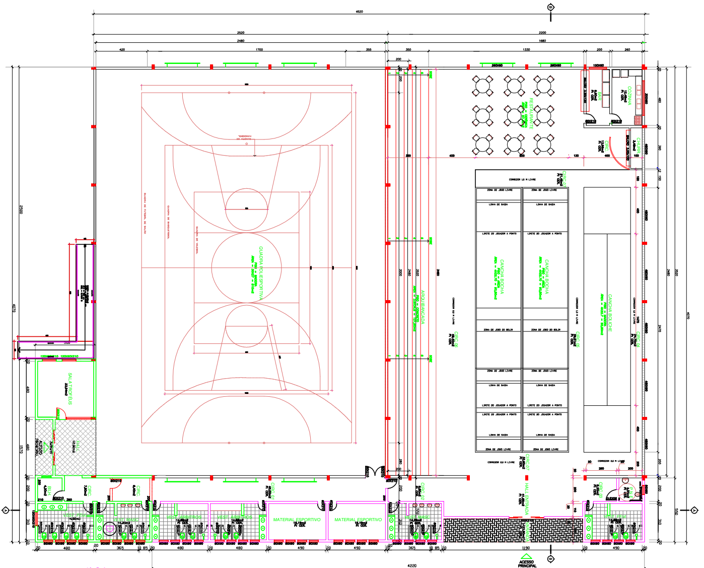
PLANTA BAIXA EXISTENTE A=1006,50 m 2
