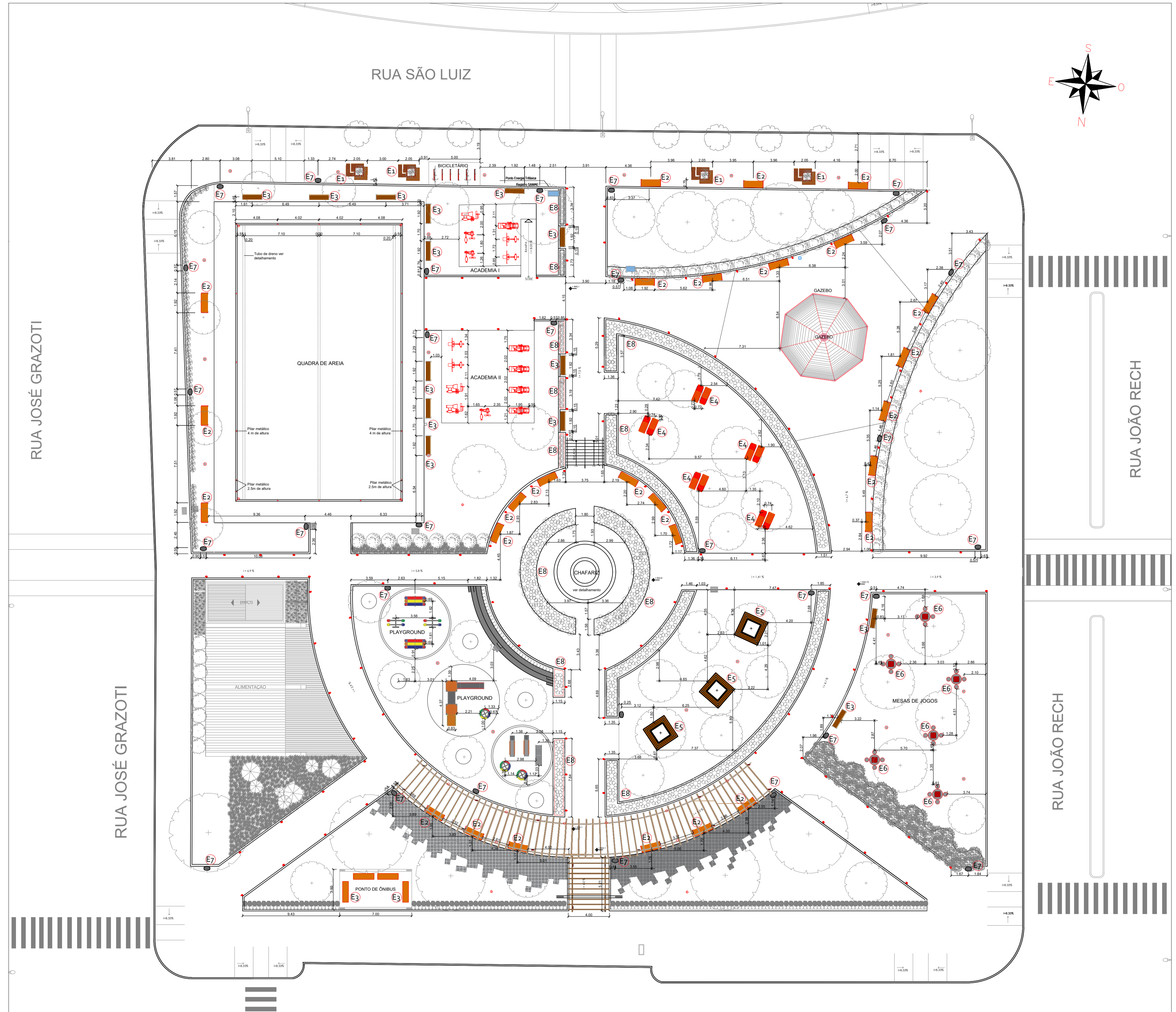
PLANTA DE MOBILIÁRIO Esc.: 1/150
