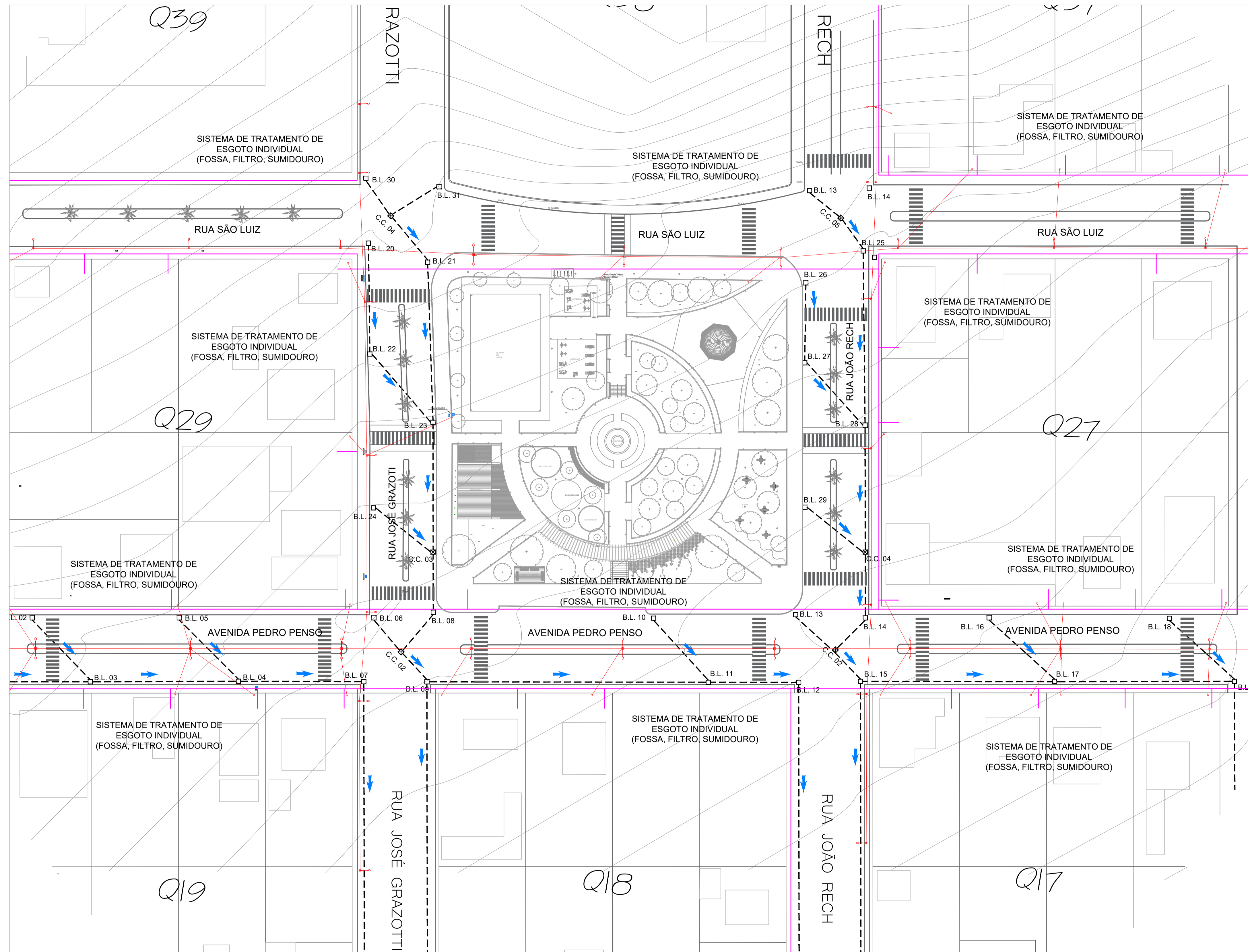
PLANTA DE INSTALAÇÕES AÉREAS E SUBTERRÂNEAS Esc.: 1/500
