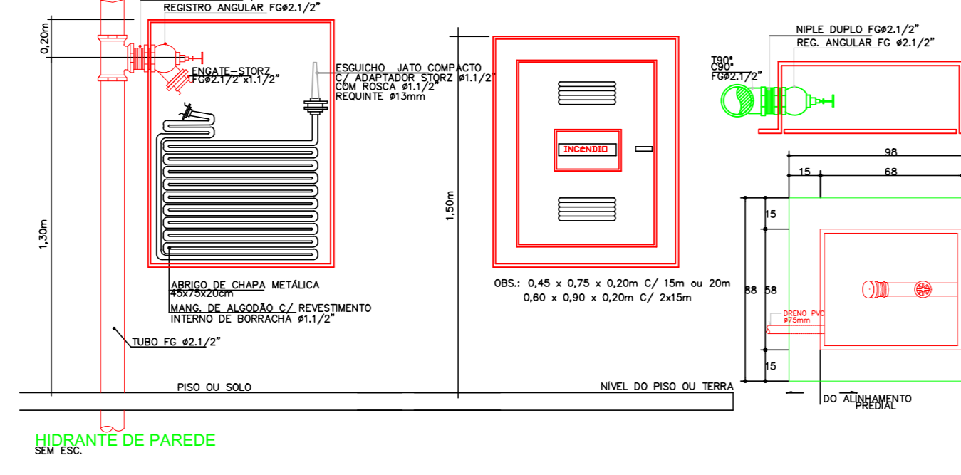
HIDRANTE DE PAREDE
