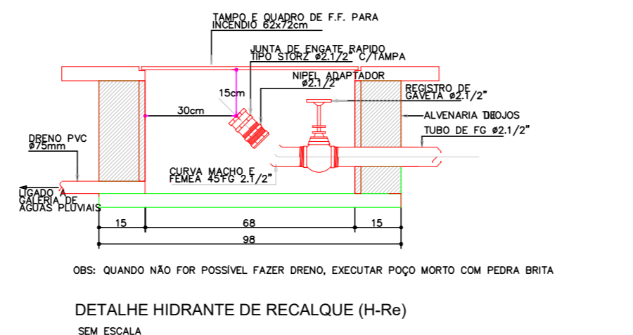
DETALHE HIDRANTE DE RECALQUE (H-Re) SEM ESCALA
