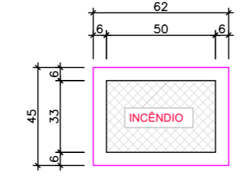
DETALHE DA TAMPA DO HIDRANTE DE RECALQUE SEM ESCALA
