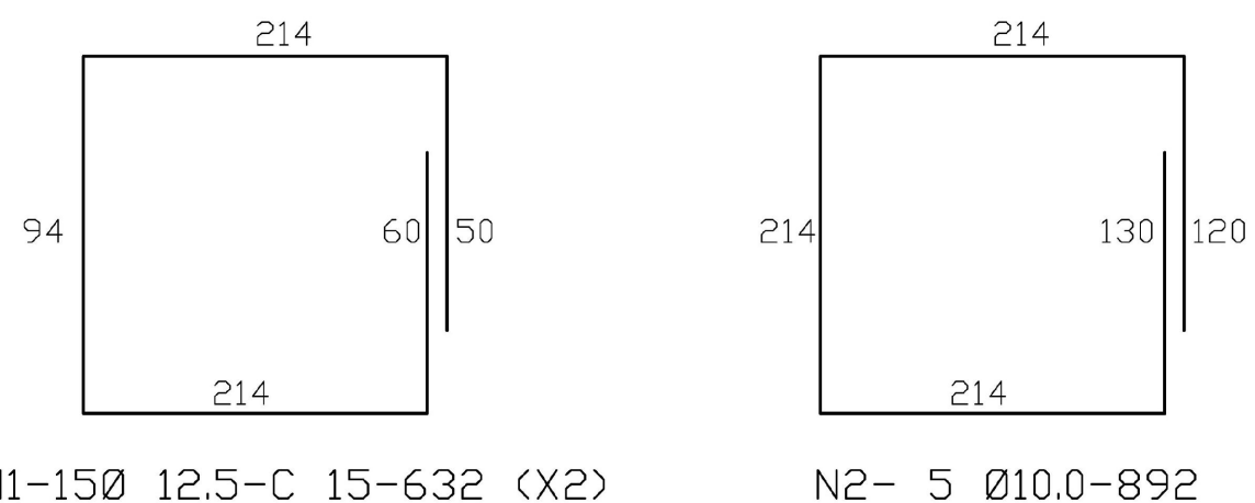
ARMADURA DO BLOCO P/ 20000L SEM ESCALA
