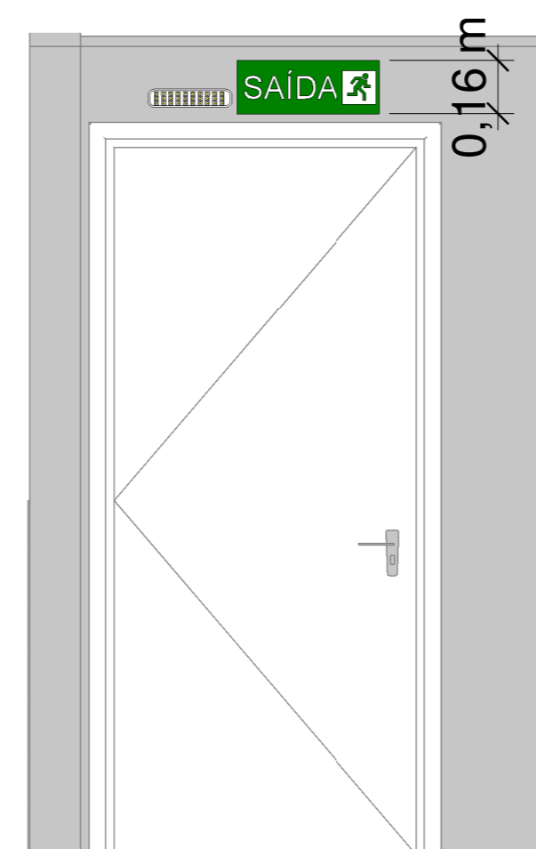
7 Detalhe - Saída de Emergência 1:20
