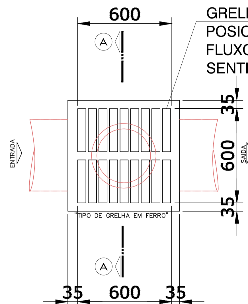
PLANTA LONGITUDINAL Sem Escala
