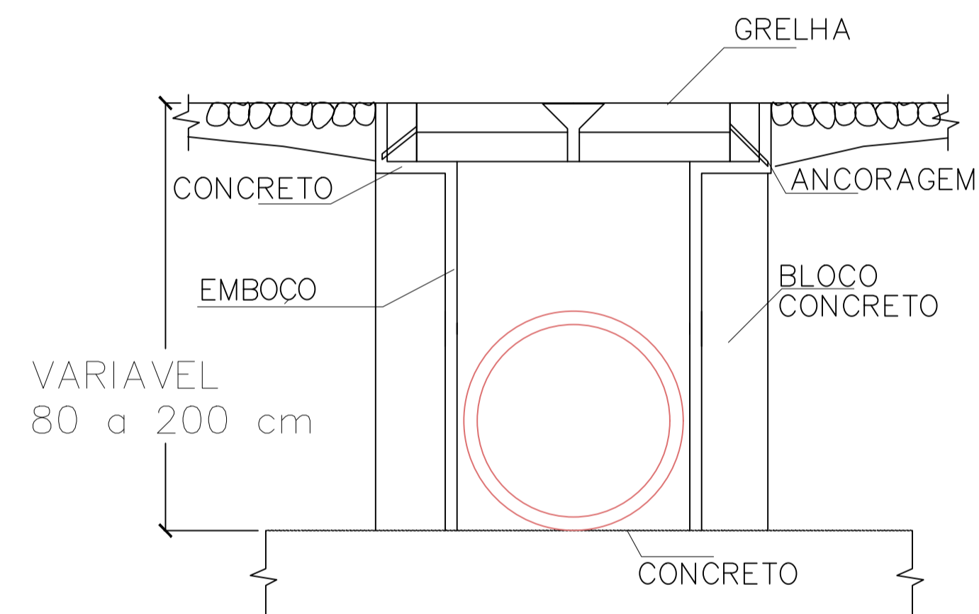
CORTE AA Sem Escala
